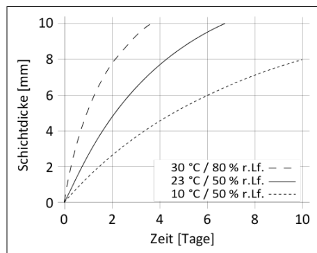
Diagramm 1: Durchhärtengeschwindigkeit Sikaflex®-268
